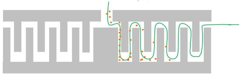
コンテナ蓋にラビリンスディスクを装着した際の断面図
